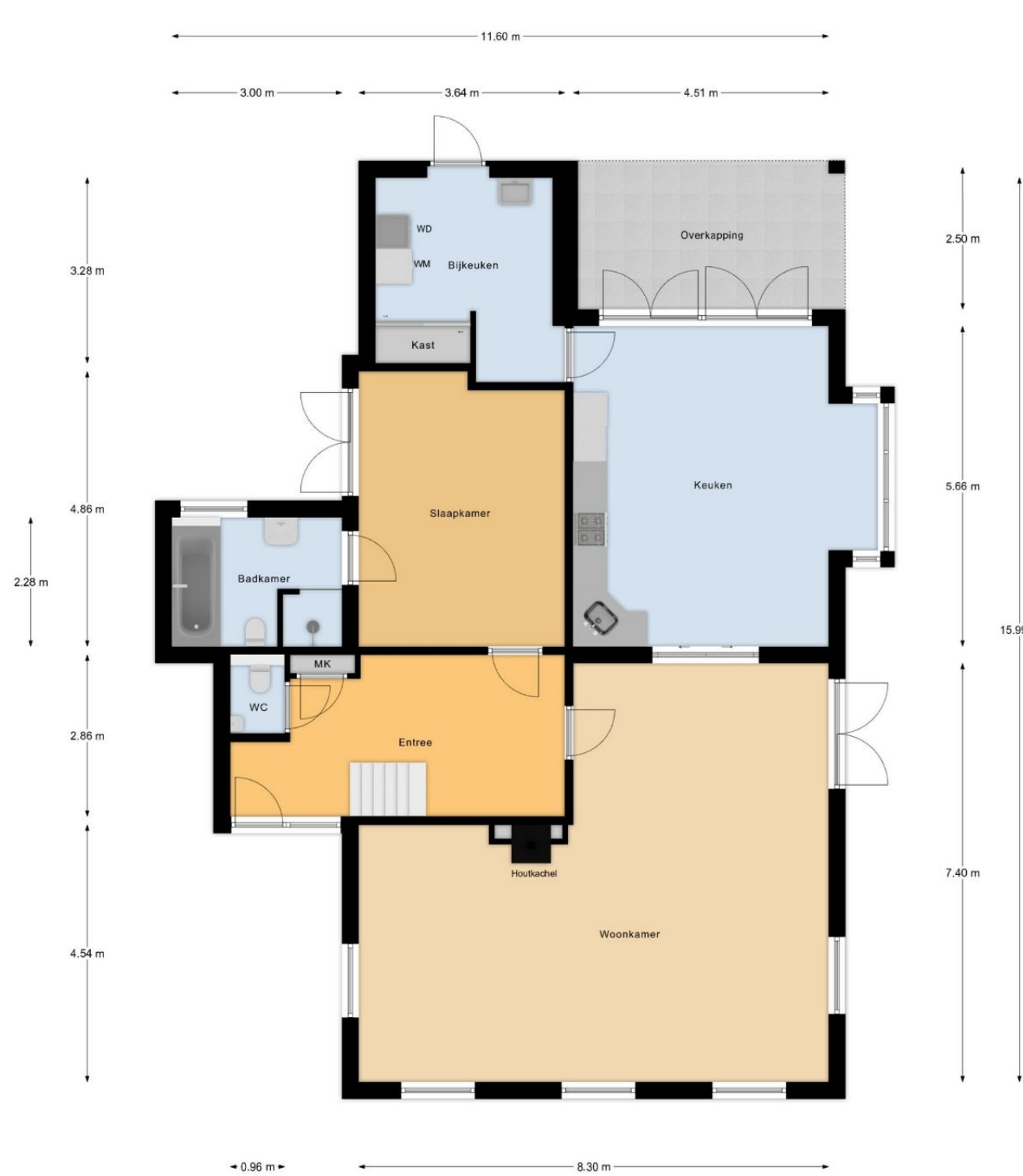
Begane Grond
